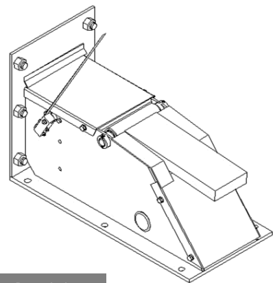
Isométrico
