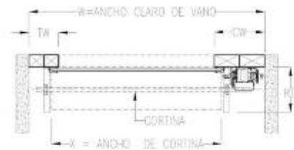
SECCIÓN A - A MONTAJE TIPO 2
